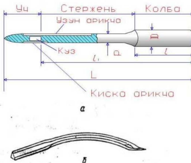
Tikuv mashinalarida ishlatiladigan igna turlari to'g'ri (a) va yoysimon (b) ignalar
